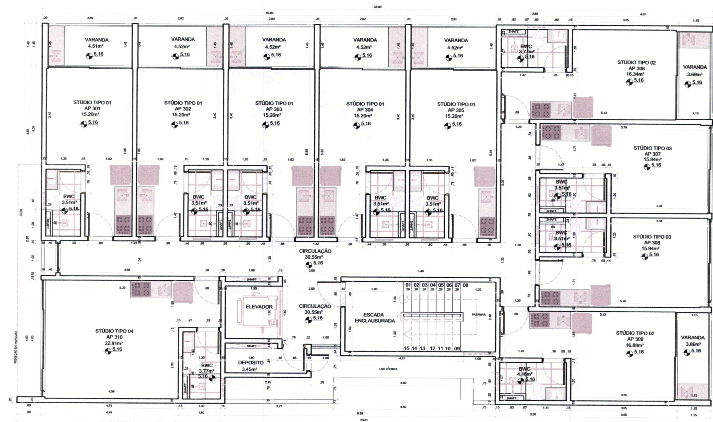
01 PLANTA BAIXA - TERCEIRO PAVIMENTO esc.: 1/75
